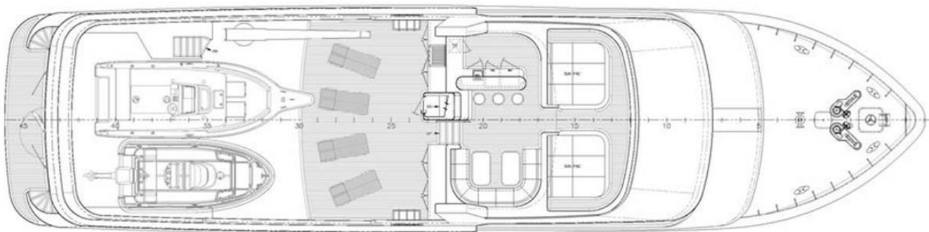
01 DECK & FLYBRIDGE
