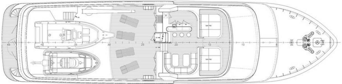
01 DECK & FLYBRIDGE
